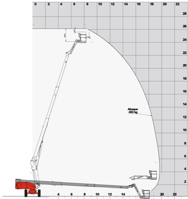
Gráfico da carga para plataforma elevatória (métrico)
